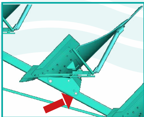
Variazione a passo in 2 pos. 2 step mechanical adjustment
