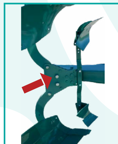
Bullone di sicurezza a taglio Shear bolt safety device
