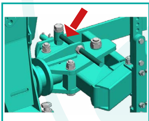
Vite per la regolazione del 1° corpo in base alla larghezza della trattore First body regulation by means of screw, according to tractor track
