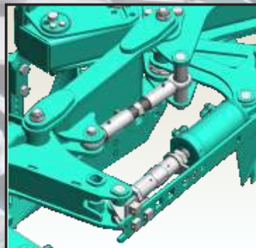
Bure spostamento del tipo scatolato chiuso e sequenza per autoallineamento al ribaltamento (di serie su 4 - 5 corpi) Box type displacement beam and sequence for selfalignment on turnover (standard on 4-5 furrows)
