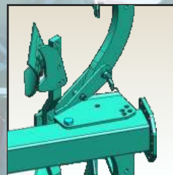
Bullone di sicurezza Shear bolt
